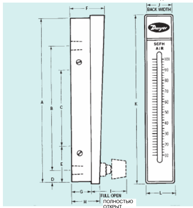
ГАБАРИТНЫЕ РАЗМЕРЫ В ДЮЙМАХ
