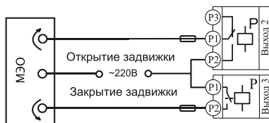
Подключение электрозадвижки
