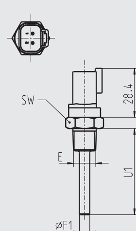
Разъём Deutsch типа DT04-2P
