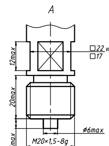
ОСЕВОЕ РАСПОЛОЖЕНИЕ ШТУЦЕРА, С ПЕРЕДНИМ ФЛАНЦЕМ
