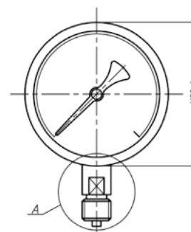
РАДИАЛЬНОЕ РАСПОЛОЖЕНИЕ ШТУЦЕРА, БЕЗ ФЛАНЦА ДЛЯ ПРИБОРОВ СО СТЕПЕНЬЮ ЗАЩИТЫ IP53
