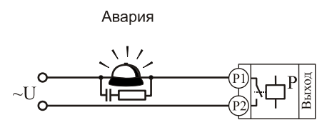
Подключение аварийной сигнализации к выходу "Р"
