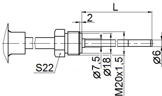
Рисунок 15 - Штуцер подвижный, кабельная погружаемая часть.
