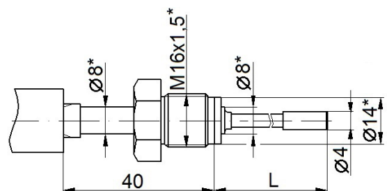
Рисунок 16 - Штуцер подвижный, кабельная погружаемая часть.
