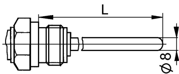
Рисунок 1 – Головка из нержавеющей стали, штуцер неподвижный
