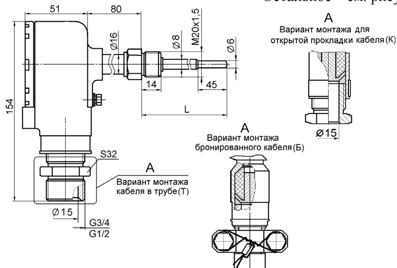
Рисунок 6 - Головка из алюминиевого сплава. Штуцер неподвижный
