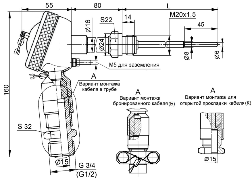
Рисунок 1 – Головка из нержавеющей стали, штуцер неподвижный
