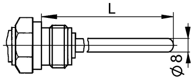
Рисунок 7 Остальное – см. рисунок 6
