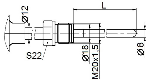
Рисунок 8 - Штуцер подвижный. Остальное – см. рисунок 6
