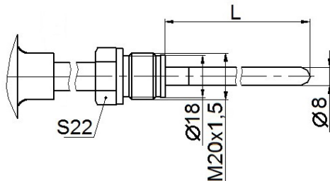
Рисунок 13 - Штуцер подвижный. Остальное – см. рисунок 11
