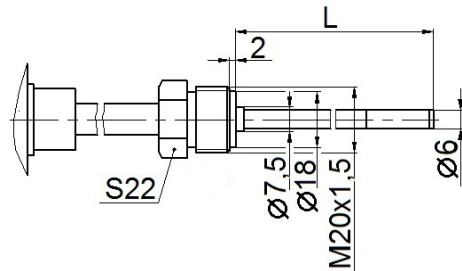
Рисунок 5 - Штуцер подвижный, кабельная погружаемая часть. Остальное – см. рисунок 1
