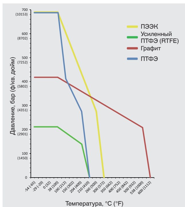
График зависимости давления от температуры
