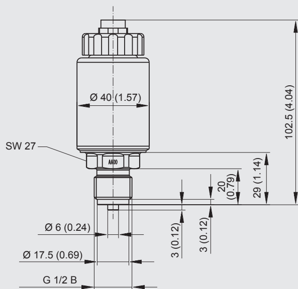
Эталонный датчик давления CPT6400
